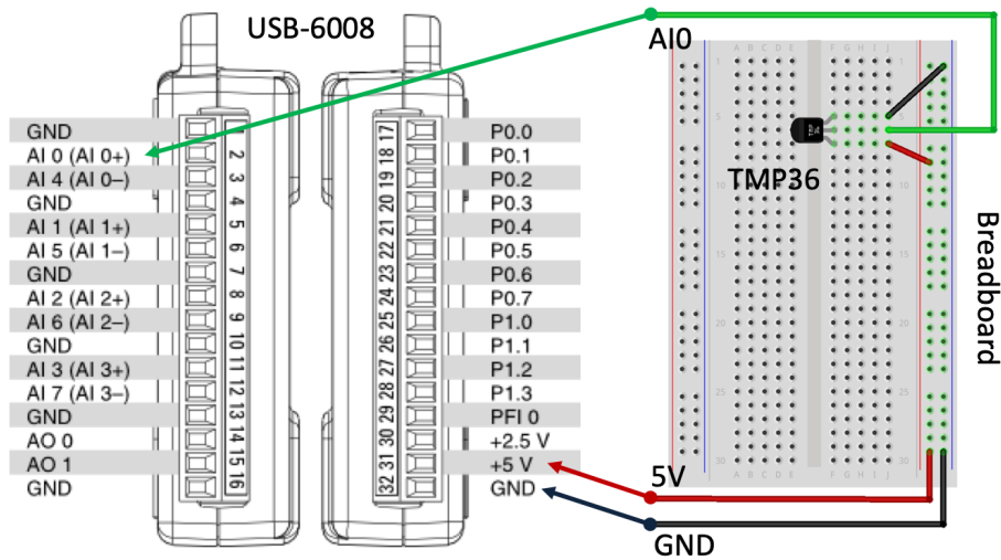
Figure 28.8: TMP36 tmp36 Wiring
